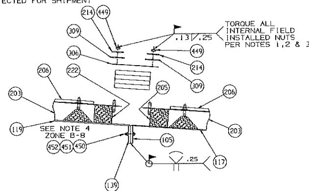
DETAIL B-5 (B-5, SH.131)
