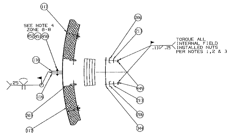
SECTION B-2 (E-4, SH.131) HORIZONTAL FIELD SPLICE TYP
