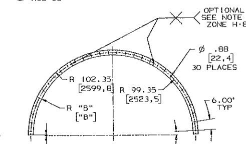
CENTER FLANGE
