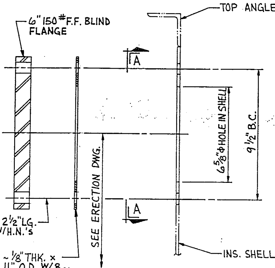
ELEVATION
